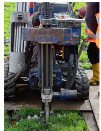
Rammsondierung
